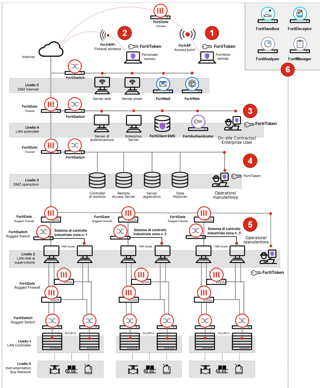
Figura 1: Accesso sicuro con le soluzioni Fortinet in un'infrastruttura IT e OT connessa
