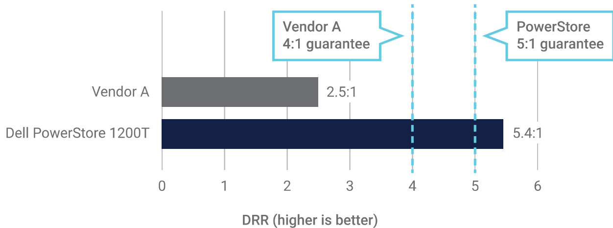
Figure 1 | Comparaison des DRR garanti et mesuré
