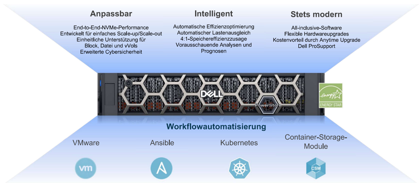
Abbildung 2. Dell PowerStore
