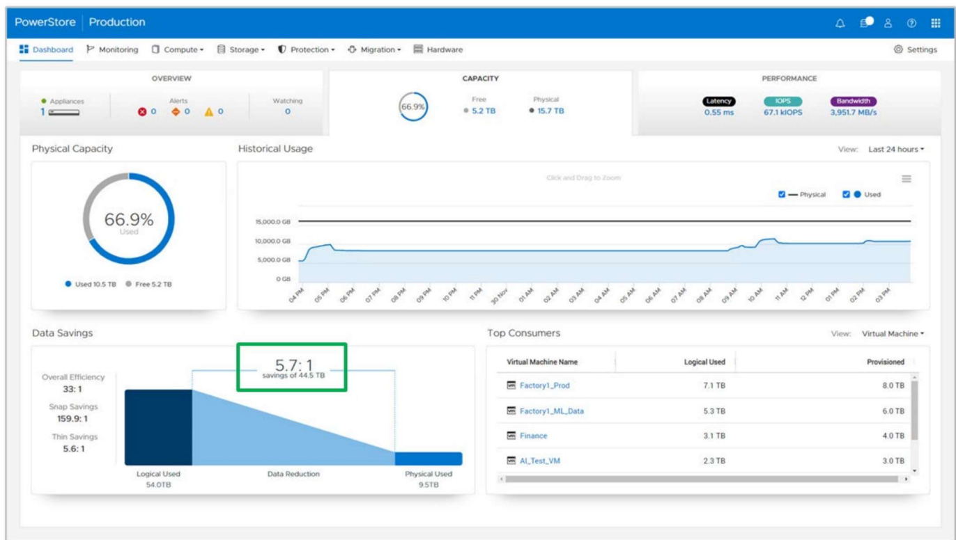
Abbildung 3. Dell PowerStore-Dashboard
