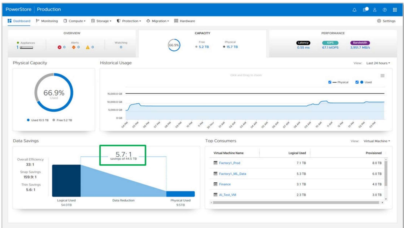
Afbeelding 3. Dell PowerStore-dashboard
